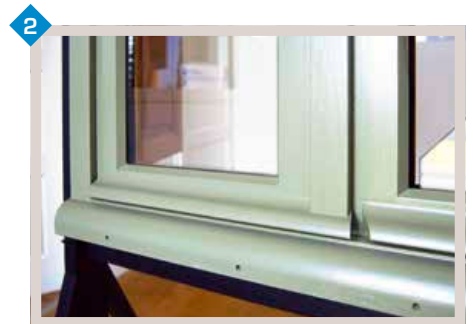
Appuis arrondis et jet d'eau à doucine
