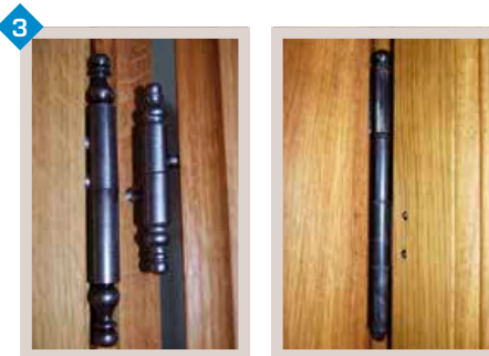
Ferrage : Fiche réglable 3D et cache-fiche de style ou Fiche à larder fer forgé à l'ancienne Crémone en fonte ou espagnolette en fer forgé, neuve ou restaurée en réemploi
